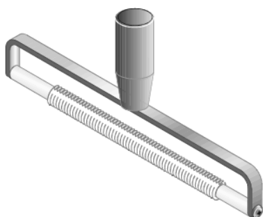
Fig. 4 Applicateur de film à spirale, modèle 358
